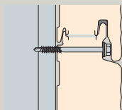
KS1000 AWP Horizontale aansluiting
