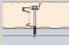
KS1000 AWP Verticale aansluiting
