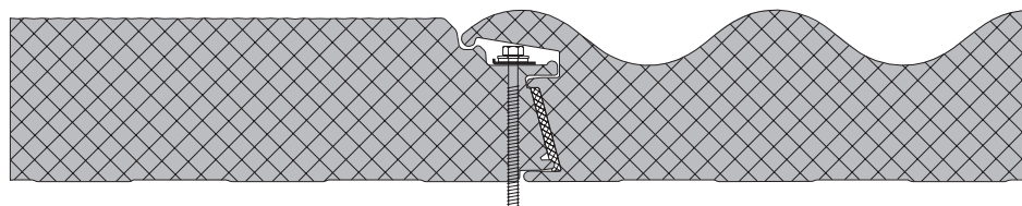
detail van de combinatie Isowand Vario® en Isowelle®
