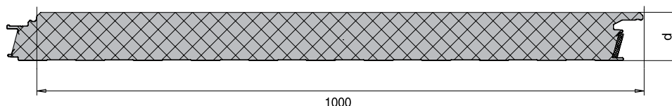
Doorsnede paneel
