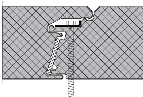
detail van een voeg Isowand Vario®
